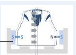
浮上・案内コイル Levitation and Guidance Coils
